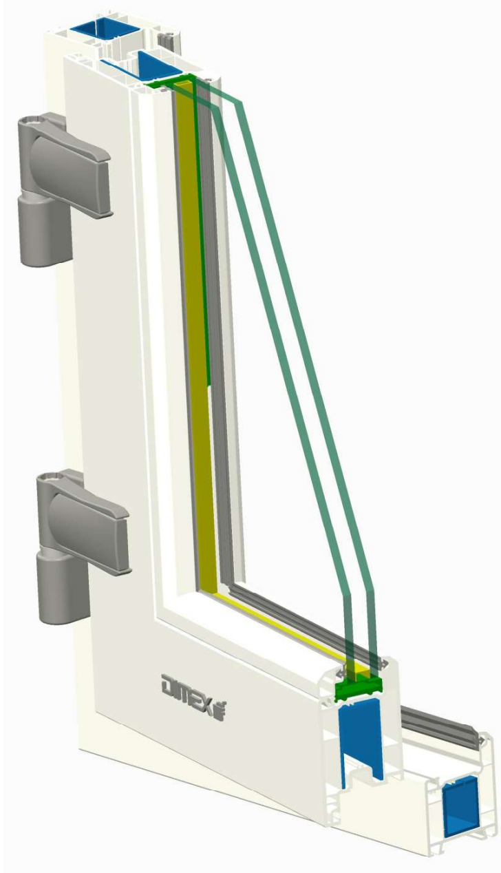
Casement Inward Opening Door Section
